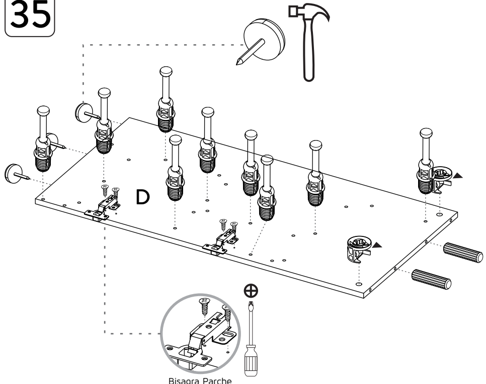
Bisagra Parche
